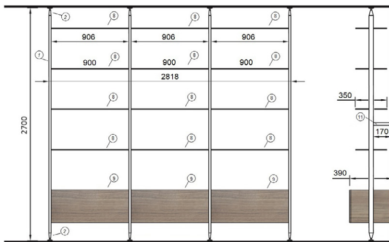
Стелажна система «ПІДЛОГА-СТЕЛЯ», специфікація для глибини каркаса 220мм і 3-х секцій по 900мм
